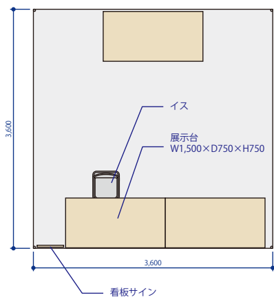
平面図
