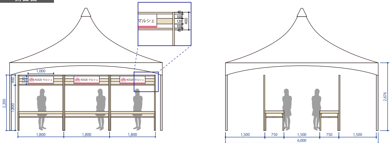
側面図
